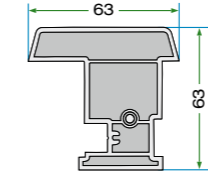
K 6023 HAREKETLİ ORTA KAYIT KAPAĞI K 6023 MOVABLE MULLION LID
