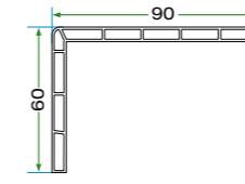
K 6024 60 x 90 PERVAZ PROFİLİ K 6024 60 x 90 BORDER PROFILE
