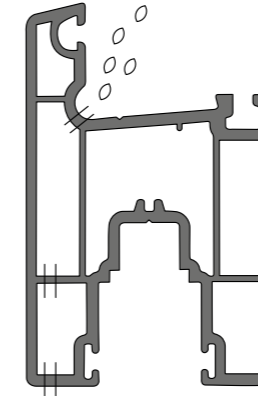
KPS 6202 Pervazlı Sürme Kanat Profili
