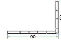
K 6024 60 x 90 PERVAZ PROFİLİ K 6024 60 x 90 BORDER PROFILE
