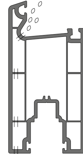
KPS 6209 Geniş Pervazlı Sürme Kanat Profili
