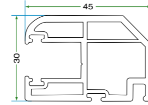
KPS 6204 SÜRME İNEKLİLİK KANAT PROFİLİ KPS 6204 FLY SCREEN SLIDING SASH PROFILE
