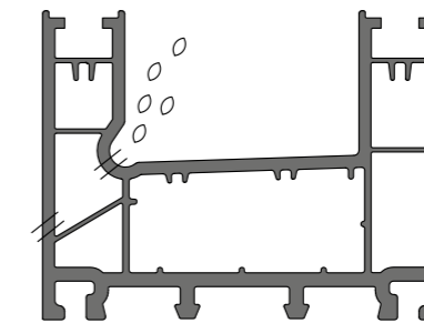
KPS 6208 Çiftli Sürme Kasa Profili
